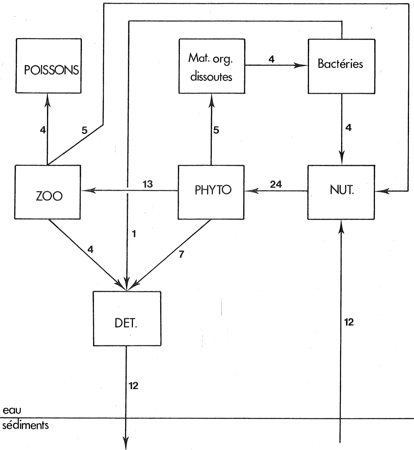
fig. 10b. Flux en g\ N/m^2.an Zone 2
